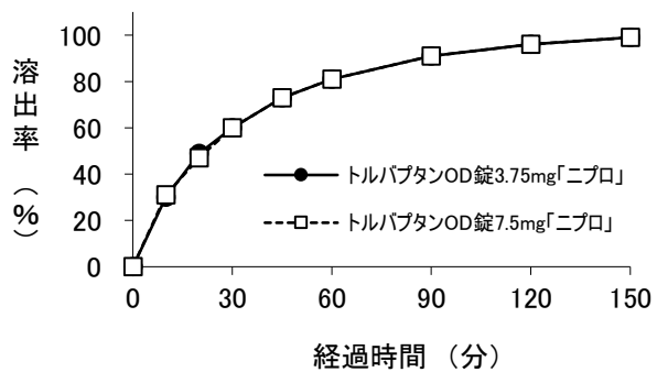
図1-5 試験液:pH 4.0 (100 rpm)
